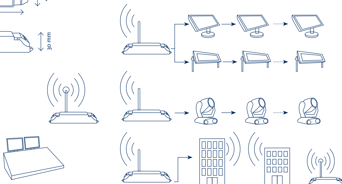
DIAGRAMA BÁSICO DE INSTALACIÓN DMX INALÁMBRICO BASIC INSTALLATION TO DMX WIRELESS
